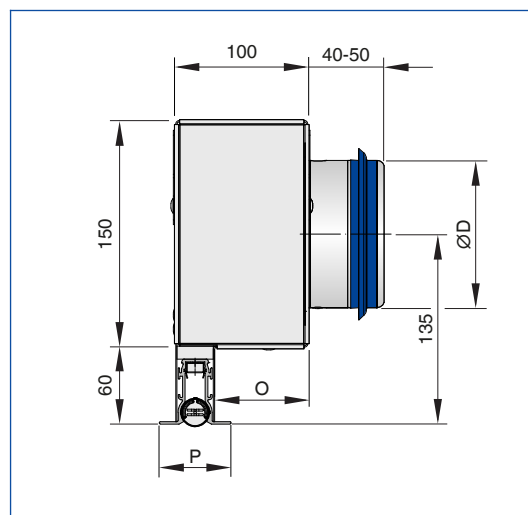
PL18-*-HA-*-B00 (асимметричное положение статической камеры, патрубков сбоку)
