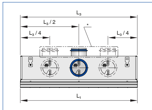
Расположение патрубка
