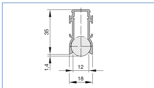
PL18-1 профиль
