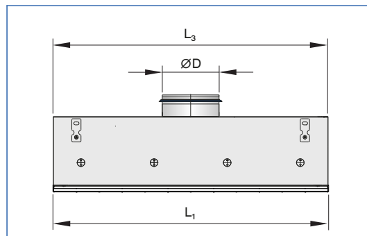
Статическая камера с патрубком сверху (VS)
