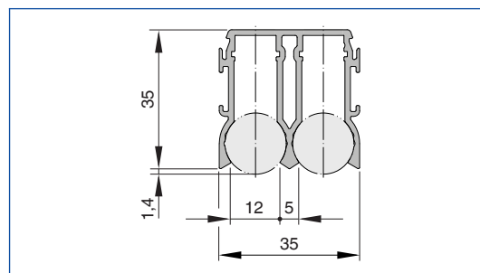
PL18-2 профиль
