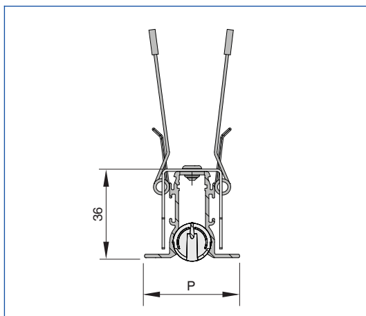
PL18-1-*-DF (лицевая панель с пружинным зажимом)
