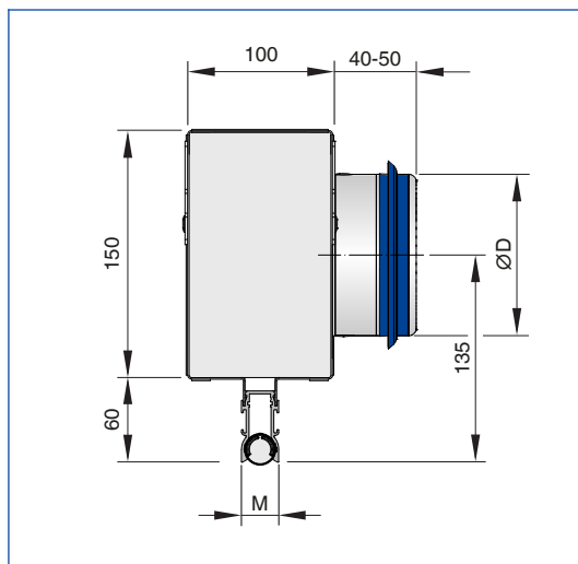
PL18-*-HS (симметричное положение статической камеры, патрубков сбоку)
