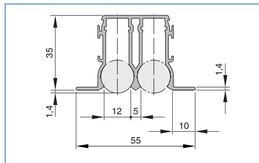
PL18-2/B00 профиль
