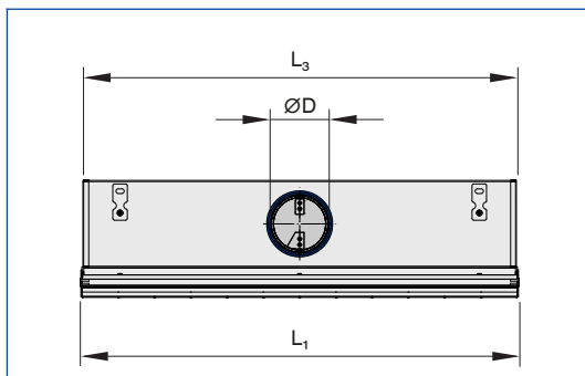
Статическая камера с патрубком сбоку (HS / HA)
