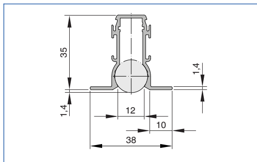
PL18-1/B00 профиль
