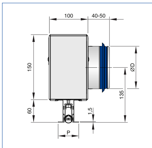
PL18-*-HS-*-B00 (симметричное положение статической камеры, патрубков сбоку)
