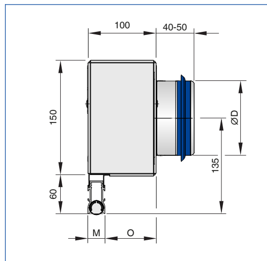
PL18-*-HA (асимметричное положение статической камеры, патрубков сбоку)
