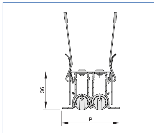
PL18-2-*-DF (лицевая панель с пружинным зажимом)
