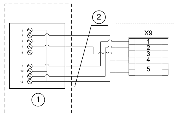
Abb. 4: Verdrahtung Raumbediengerät Thermokon an Klemme X9
