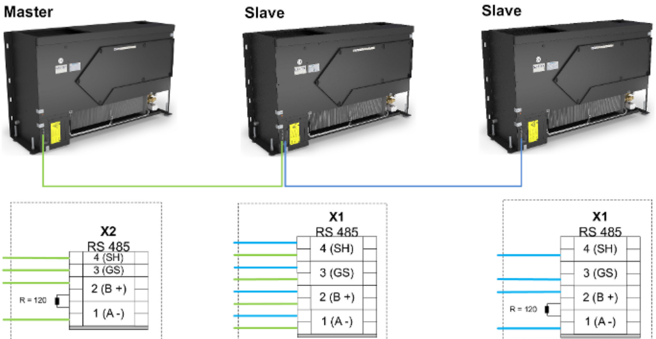
Abb. 11: FSL-CONTROL III Kommunikation 3 Geräte
