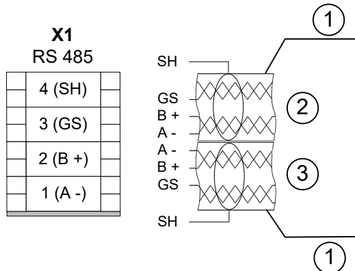
Abb. 15: Anschluss MBE/GA an Master-Gerät mit Modbus RTU / BACnet MS/TP Schnittstelle
