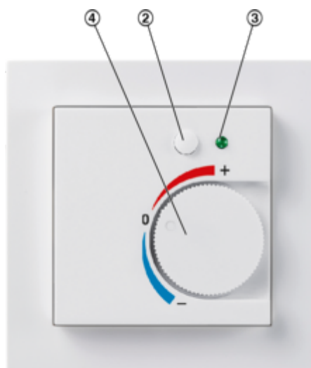
Abb. 34: Raumbediengerät ohne Stufenschalter, Unterputzmontage, passend zu Schalterprogramm Gira E2, FSL-CONTROL III, Artikelnummer: A0000082916
