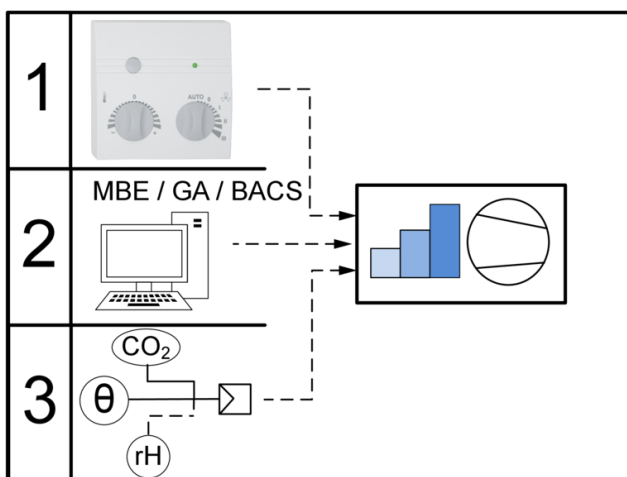
Abb. 22: Prioritäten Ventilatorstufenschaltung
