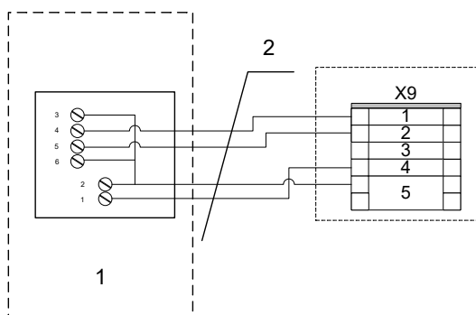
Abb. 6: Verdrahtung Raumbediengerät Thermokon an Klemme X9
