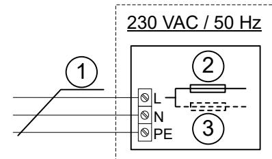
Abb. 1: Anschluss Versorgungsspannung
