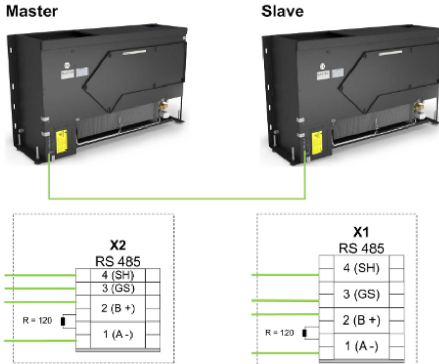
Abb. 10: FSL-CONTROL III Kommunikation 2 Geräte
