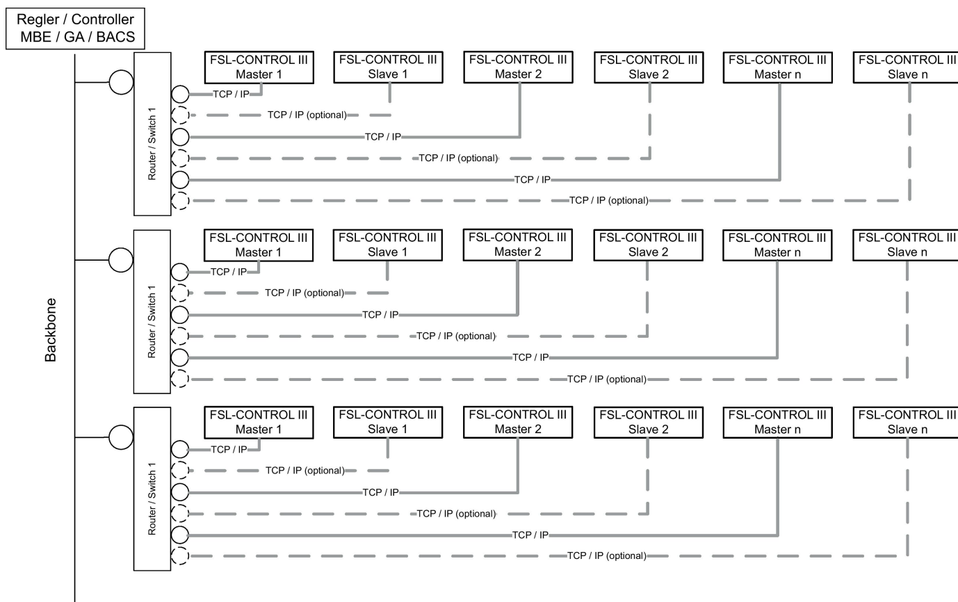
Abb. 14: FSL-CONTROL III Netzwerkaufbau, Modbus TCP; BACnet IP
