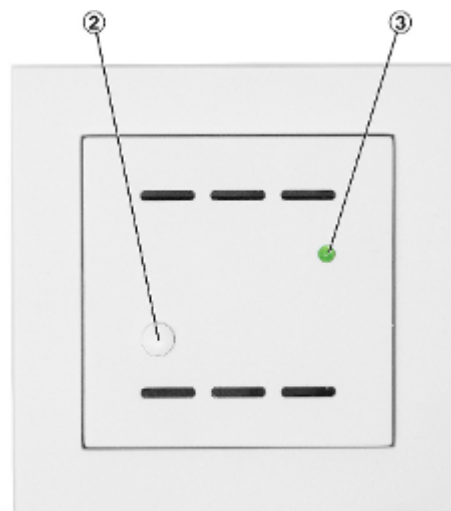
Abb. 35: Raumbediengerät ohne Stufenschalter und ohne Sollwertsteller für Unterputzmontage, passend zu Schalterprogramm Gira E2, Typ WRF06-TD-NTC20k, Artikelnummer: A0000081503
