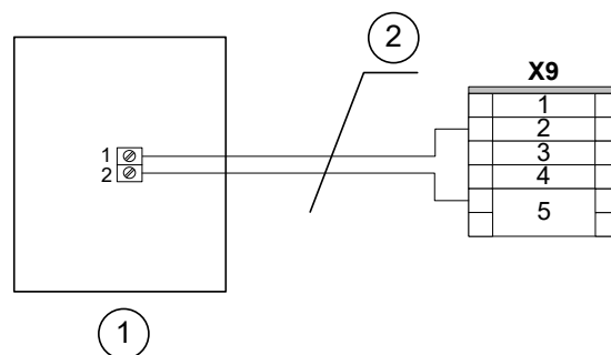
Abb. 7: Anschluss Raumtemperaturfühler
