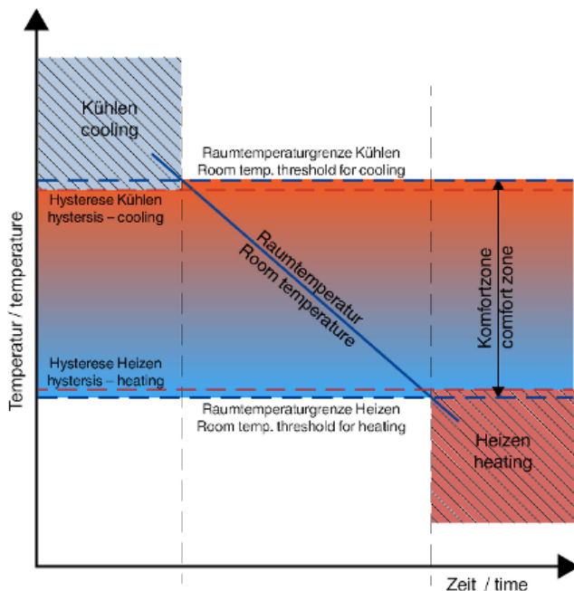
Abb. 21: Raumtemperaturregelung
