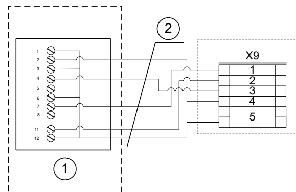
Abb. 3: Verdrahtung Raumbediengerät Thermokon, 5-stufig an Klemme X9
