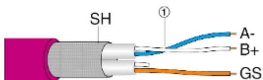
Abb. 12: Verdrahtung
