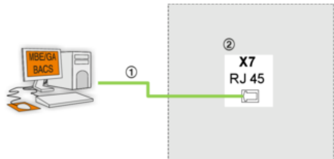
Abb. 17: Anschluss MBE/GA an Master-Gerät mit Modbus TCP / BACnet IP Schnittstelle
