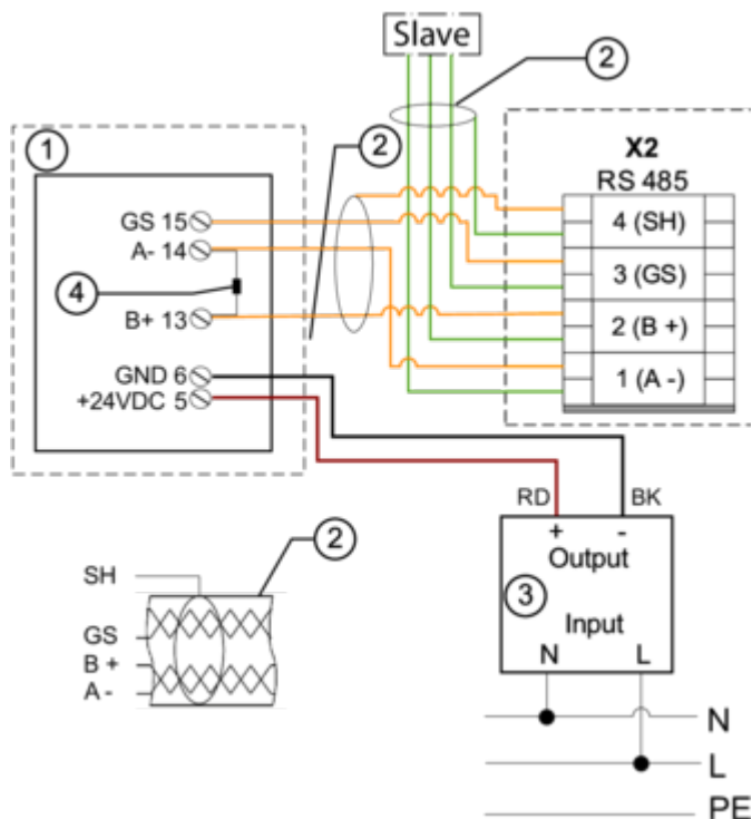
Abb. 2: Verdrahtung digitales Raumbediengerät Typ Schneider an Klemme X2
