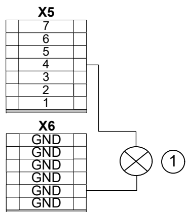
Abb. 54: Anschlussbeispiel B-Alarm
