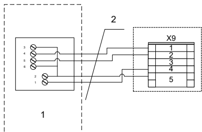
Abb. 52: Verdrahtung Raumbediengerät Thermokon an Klemme X9
