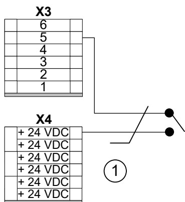
Abb. 53: Anschlussbeispiel Fensterkontakt
