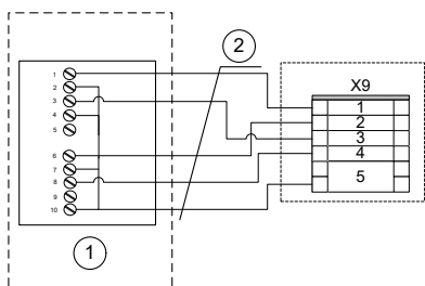
Abb. 51: Verdrahtung Raumbediengerät Thermokon an Klemme X9
