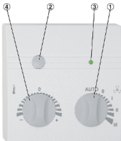
Abb. 71: Raumbediengerät mit Stufenschalter, für Aufputzmontage Typ WRF04 PSTD NTC20k 5k FS5 gn 5V SA Artikelnummer: A00000082515
