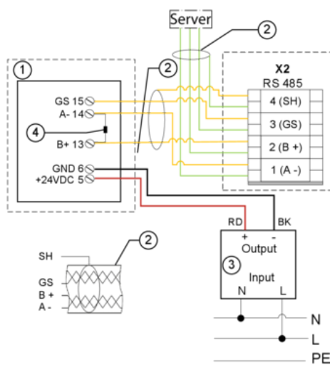
Abb. 48: Verdrahtung digitales Raumbediengerät Typ Schneider an Klemme X2
