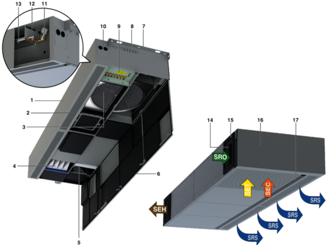
Abb. 2: Lüftungsgerät SCHOOLAIR-D-HV
