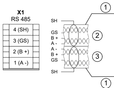
Abb. 59: Anschluss MBE/GA an Master-Gerät mit Modbus RTU
