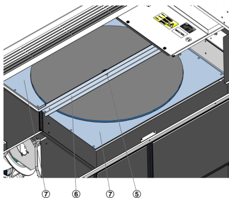
Abb. 92: RWT-Gehäuse öffnen
