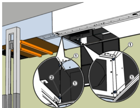
Abb. 14: Bauteil 2 neben Bauteil 1 positionieren
