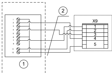
Abb. 49: Verdrahtung Raumbediengerät Thermokon, 5-stufig an Klemme X9
