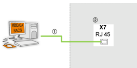
Abb. 58: Anschluss MBE/GA an Master-Gerät mit Modbus TCP / BACnet IP
