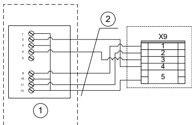
Abb. 50: Verdrahtung Raumbediengerät Thermokon an Klemme X9
