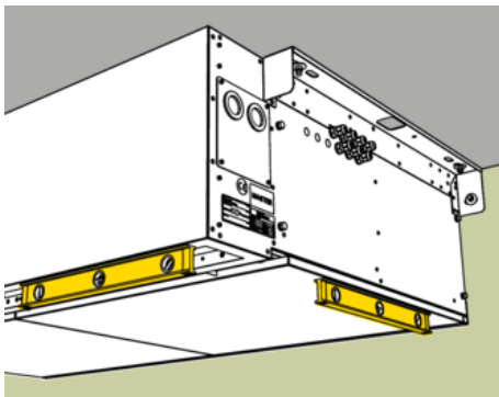
Abb. 11: SA-D-HV-ausrichten
