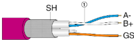
Abb. 57: Verdrahtung
