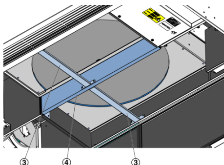
Abb. 91: Kammerblech und Streben
