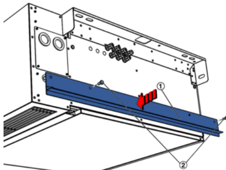
Abb. 21: Deckenanschluss-Schiene befestigen
