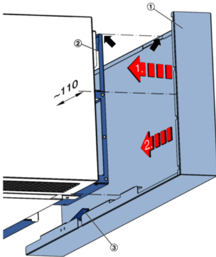
Abb. 23: Abdeckung aufschieben
