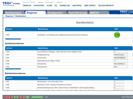
Abb. 69: Webvisualisierung Geräteseite
