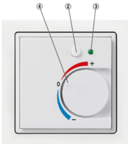
Abb. 74: Raumbediengerät ohne Stufenschalter, für Unterputzmontage passend zu Schalterprogramm Busch Jäger Future linear Typ: WRF07 PTD NTC20k BType6 5k gn, Artikelnummer: A00000079779
