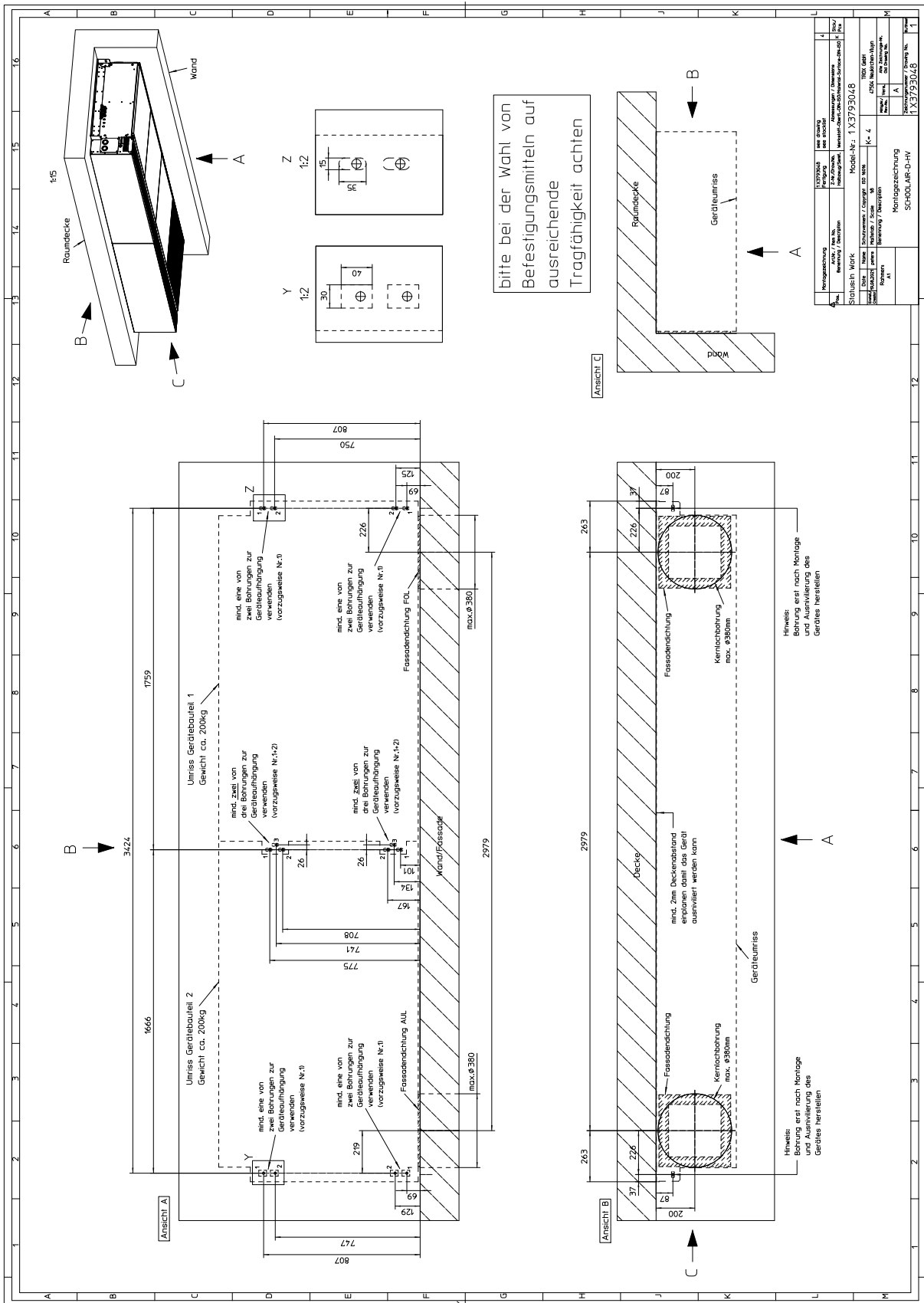
Abb. 97: SA-D-HV Montagezeichnung
