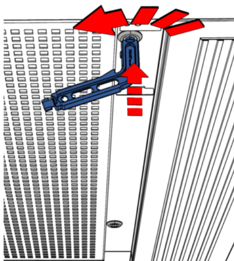
Abb. 80: Revisionsdeckel-Verschluss öffnen
