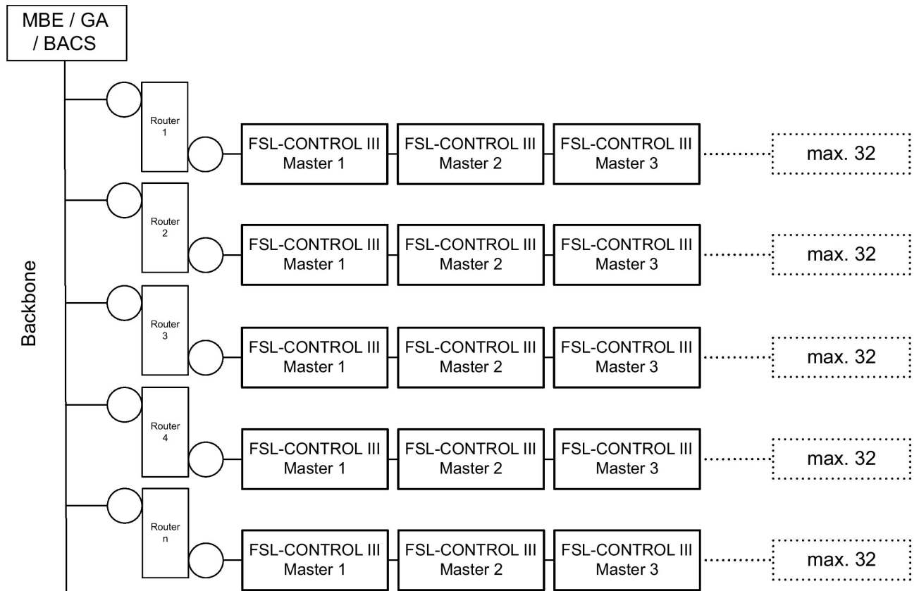
Abb. 61: FSL-CONTROL III Netzwerkaufbau, Beispiel Modbus RTU; BACnet MS/TP
