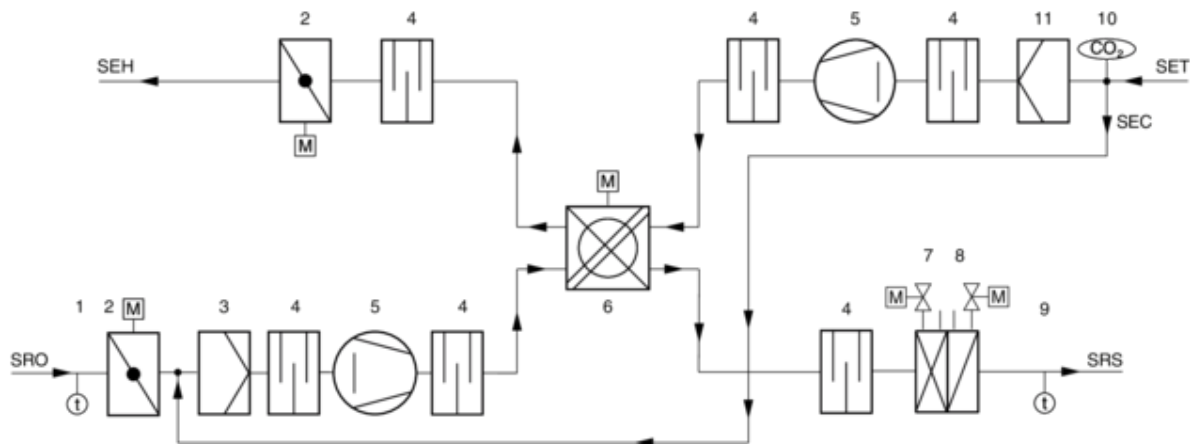
Abb. 3: Lüftungsschema SCHOOLAIR-D-HV
