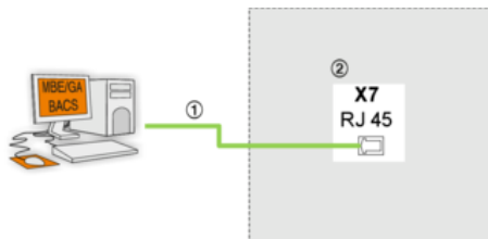
Abb. 60: Anschluss MBE/GA an Slave-Gerät mit Modbus TCP
