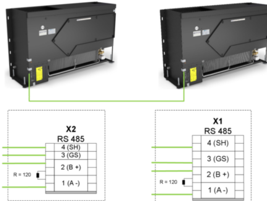
Abb. 55: FSL-CONTROL III Kommunikation 2 Geräte
