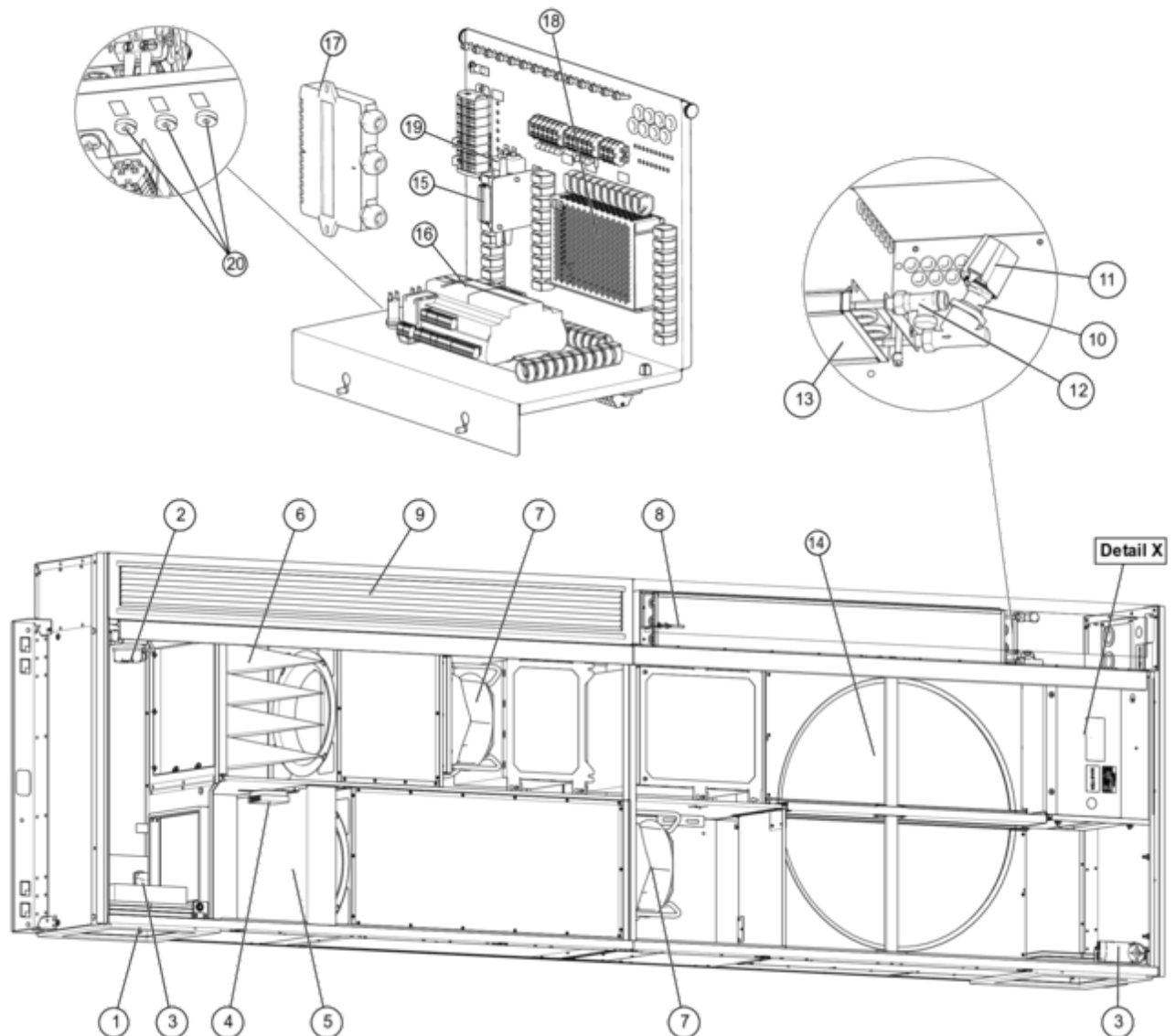
Abb. 96: SCHOOLAIR-D-HV Ersatzteile
