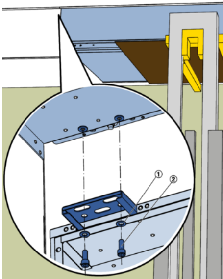
Abb. 39: Bauteil 1 in die Zarge einsetzen und verschrauben
