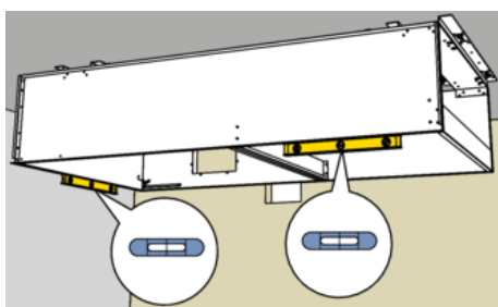
Abb. 27: SA-D-HV-ausrichten
