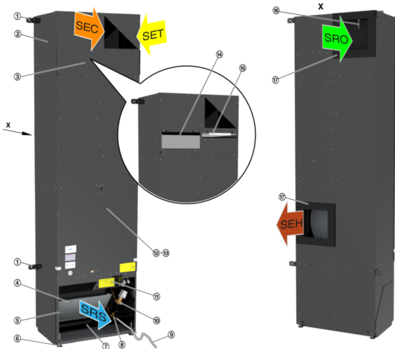
Abb. 2: Lüftungsgerät SCHOOLAIR-V-HV
