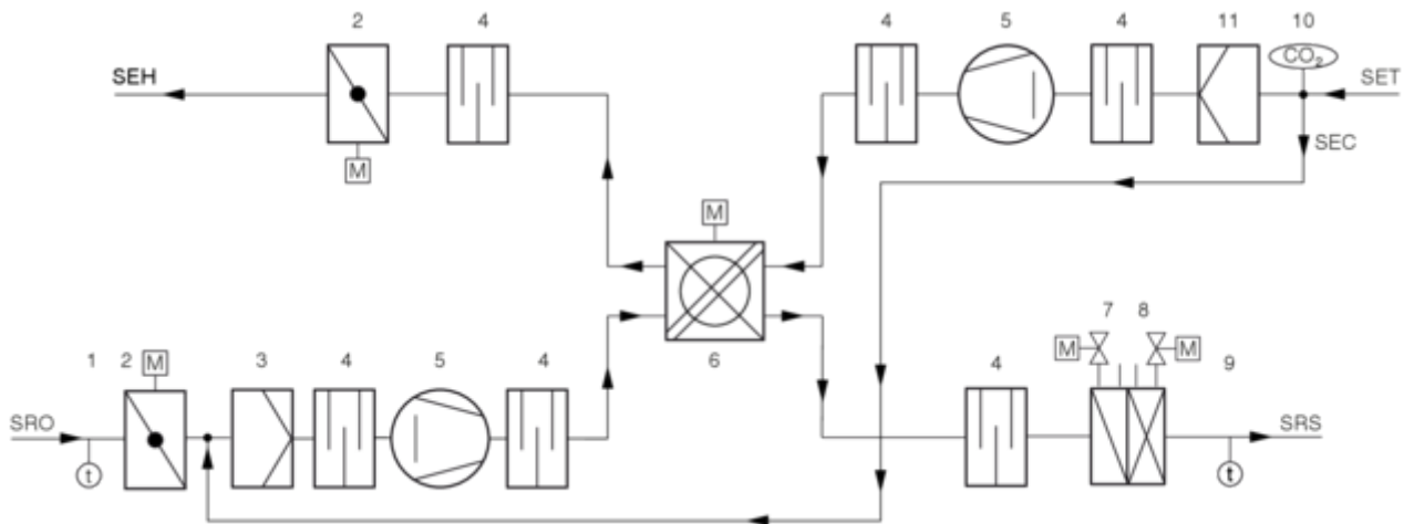
Abb. 3: Lüftungsschema SCHOOLAIR-V-HV
