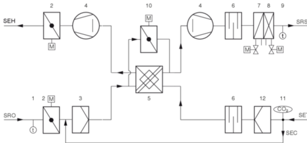
Abb. 3: Lüftungsschema SCHOOLAIR-V-1800
