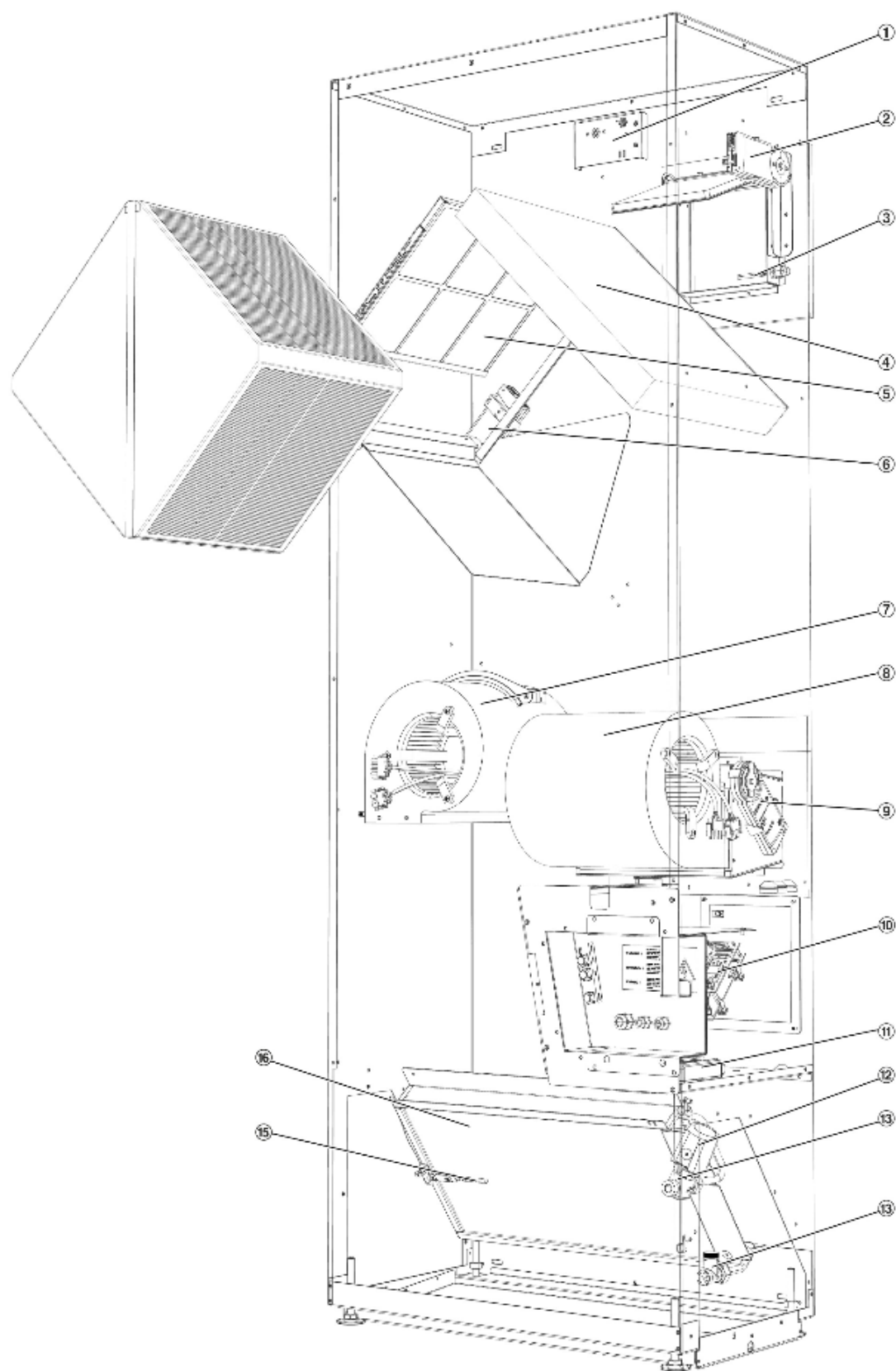
Abb. 42: Ersatzteile SCHOOLAIR-V-1800, Wärmerückgewinner herausgezogen
