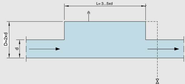
Abb. 34: Luftabscheider mit Querschnittsvergrößerung
