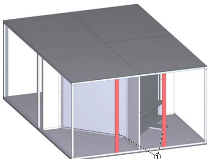
Abb. 18: Montage vorbereiten
