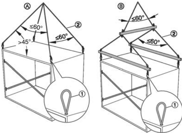
Abb. 6: Krantransport an Seilösen
