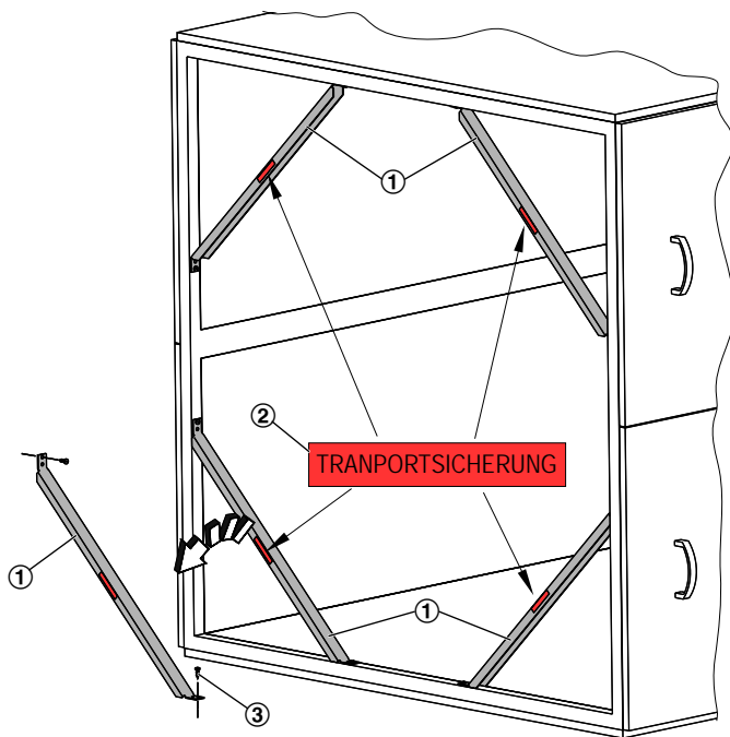
Abb. 10: Transportsicherung mit Traversen
