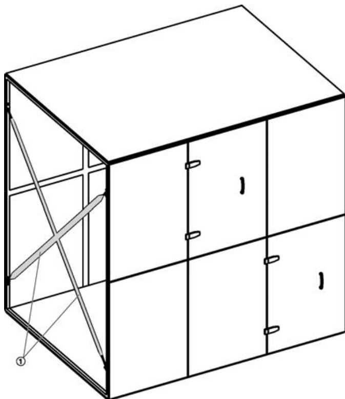
Abb. 5: Verstrebungen
