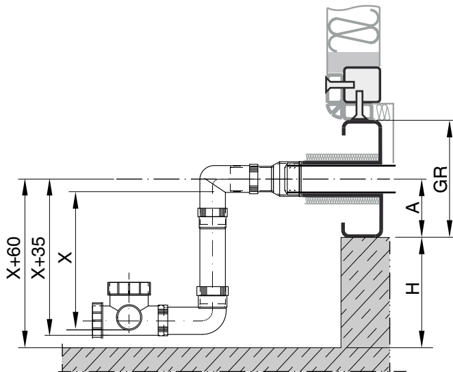
Abb. 28: Siphon für Unterdruck
