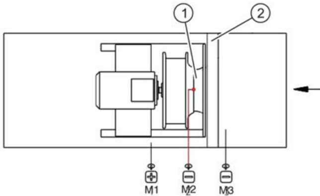
Abb. 43: Druckmessstelle
