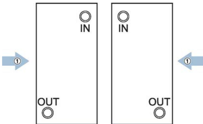
Abb. 35: Beispielhafte Darstellung der Dampfwärmeübertrageranschlüsse im Gegenstrom
