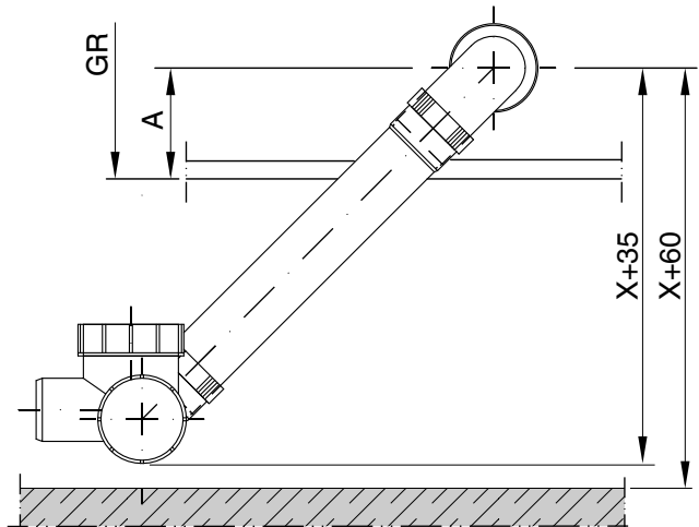
Abb. 31: Schrägstellung bei Unterdruck Siphon
