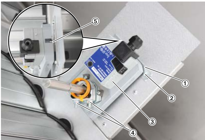
Abb. 20: Stellantrieb montieren
