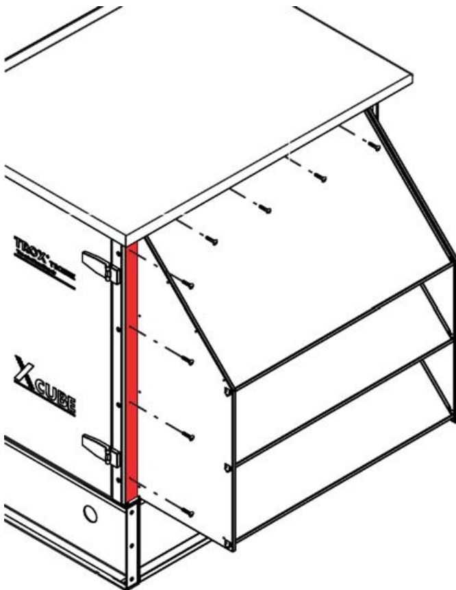
Abb. 25: Wetterschutzhaube anschrauben
