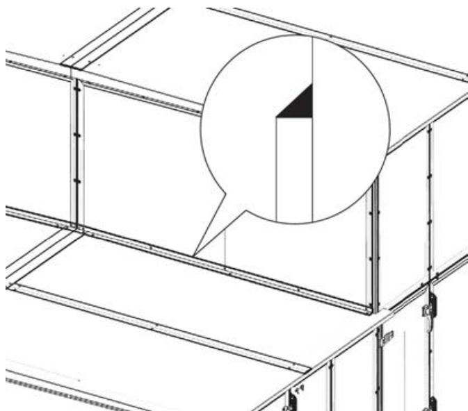
Abb. 23: Höhenversatz
