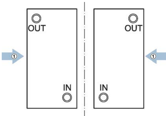
Abb. 32: Beispielhafte Darstellung der Wärmeübertragerschlüsse im Gegenstrom
