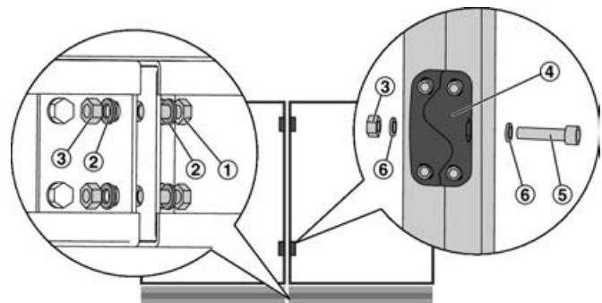
Abb. 16: Grundrahmen verschrauben
