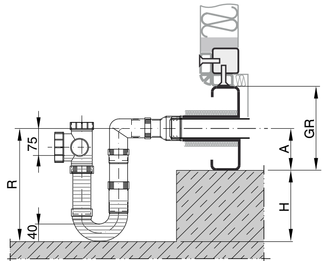
Abb. 29: Siphon Überdruck
