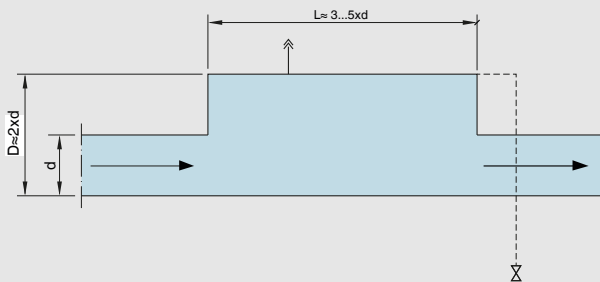
Abb. 38: Luftabscheider mit Querschnittsvergrößerung
