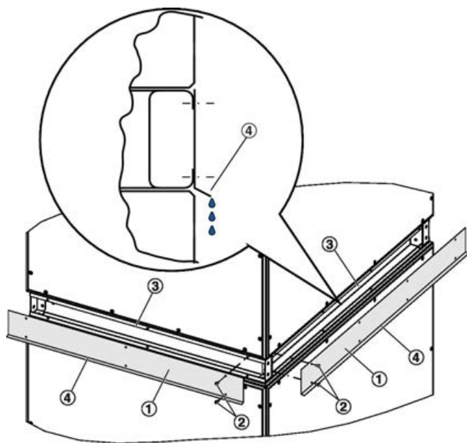
Abb. 27: Abdeckung montieren
