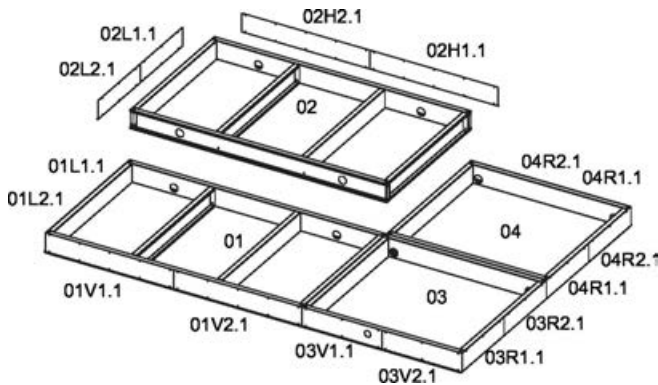
Abb. 26: Kennzeichnung der Grundrahmenabdeckungen
