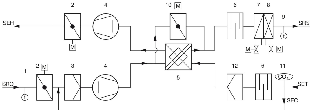
Abb. 3: Lüftungsschema SCHOOLAIR-B
