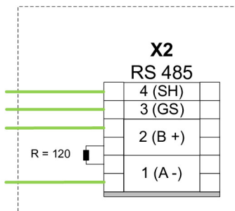
Abb. 12: FSL-CONTROL III Kommunikation 2 Geräte
