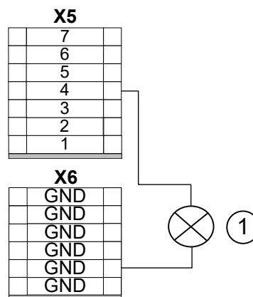
Abb. 11: Anschlussbeispiel B-Alarm
