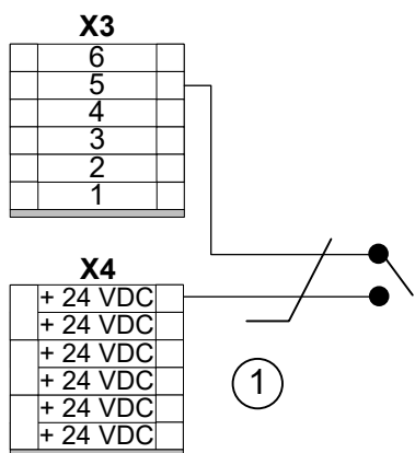
Abb. 10: Anschlussbeispiel Fensterkontakt
