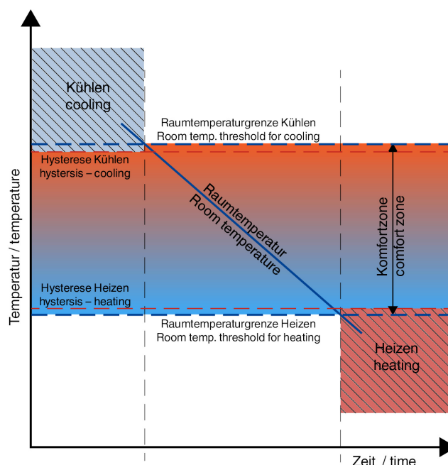
Abb. 21: Raumtemperaturregelung
