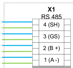
Abb. 13: FSL-CONTROL III Kommunikation 3 Geräte
