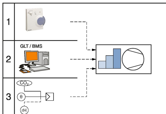
Abb. 22: Prioritäten Ventilatorstufenschaltung
