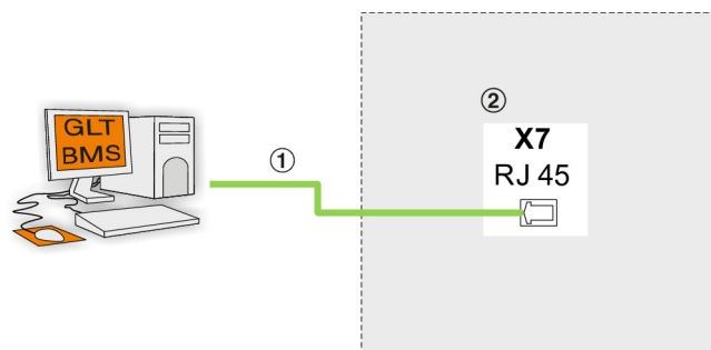
Abb. 18: Anschluss GLT an Master-Gerät mit Modbus TCP / BACnet IP Schnittstelle
