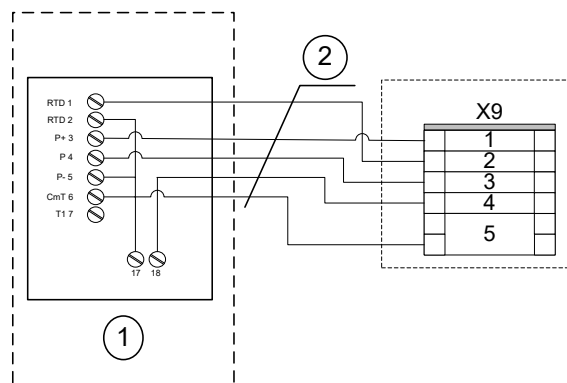
Abb. 4: Verdrahtung Raumbediengerät Titec RTF3-NTC20k-P5k-T-L an Klemme X9
