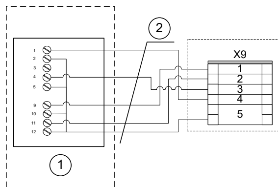
Abb. 5: Verdrahtung Raumbediengerät Thermokon an Klemme X9
