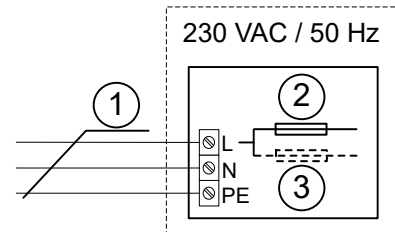
Abb. 1: Anschluss Versorgungsspannung
