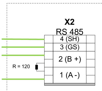
Abb. 13: FSL-CONTROL III Kommunikation 3 Geräte
