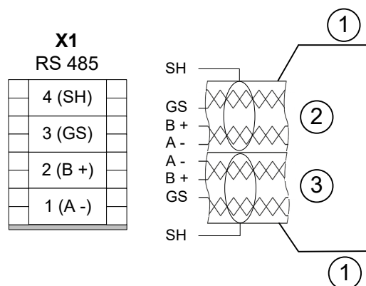
Abb. 19: Anschluss MBE / GA an Master-Gerät mit Modbus RTU
