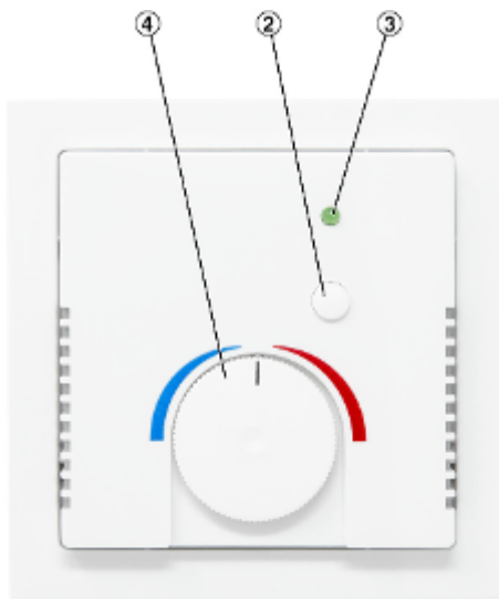
Abb. 34: Raumbediengerät ohne Stufenschalter, für Unterputzmontage passend zu Schalterprogramm Busch Jäger Future linear Typ: WRF07 PTD NTC20k BType6 5k gn, Artikelnummer: A0000079779
