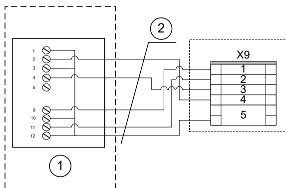
Abb. 10: Verdrahtung Raumbediengerät Thermokon an Klemme X9
