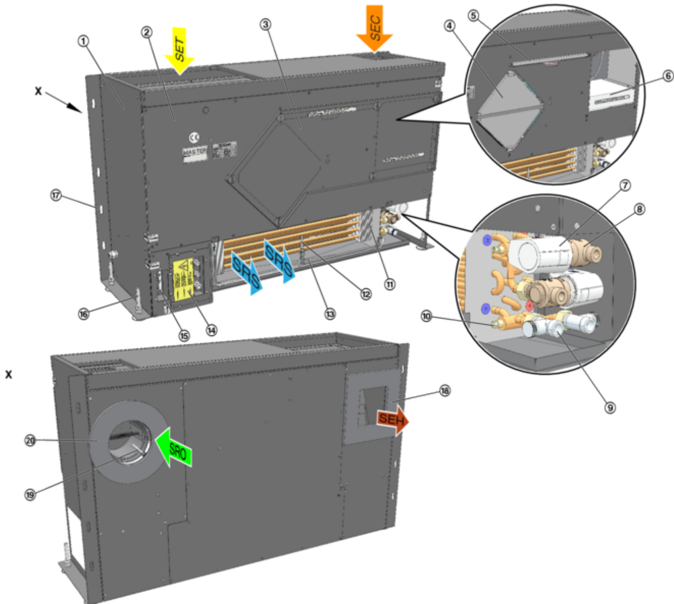
Abb. 2: Lüftungsgerät ROOMAIR-B-ZAB/SEK
