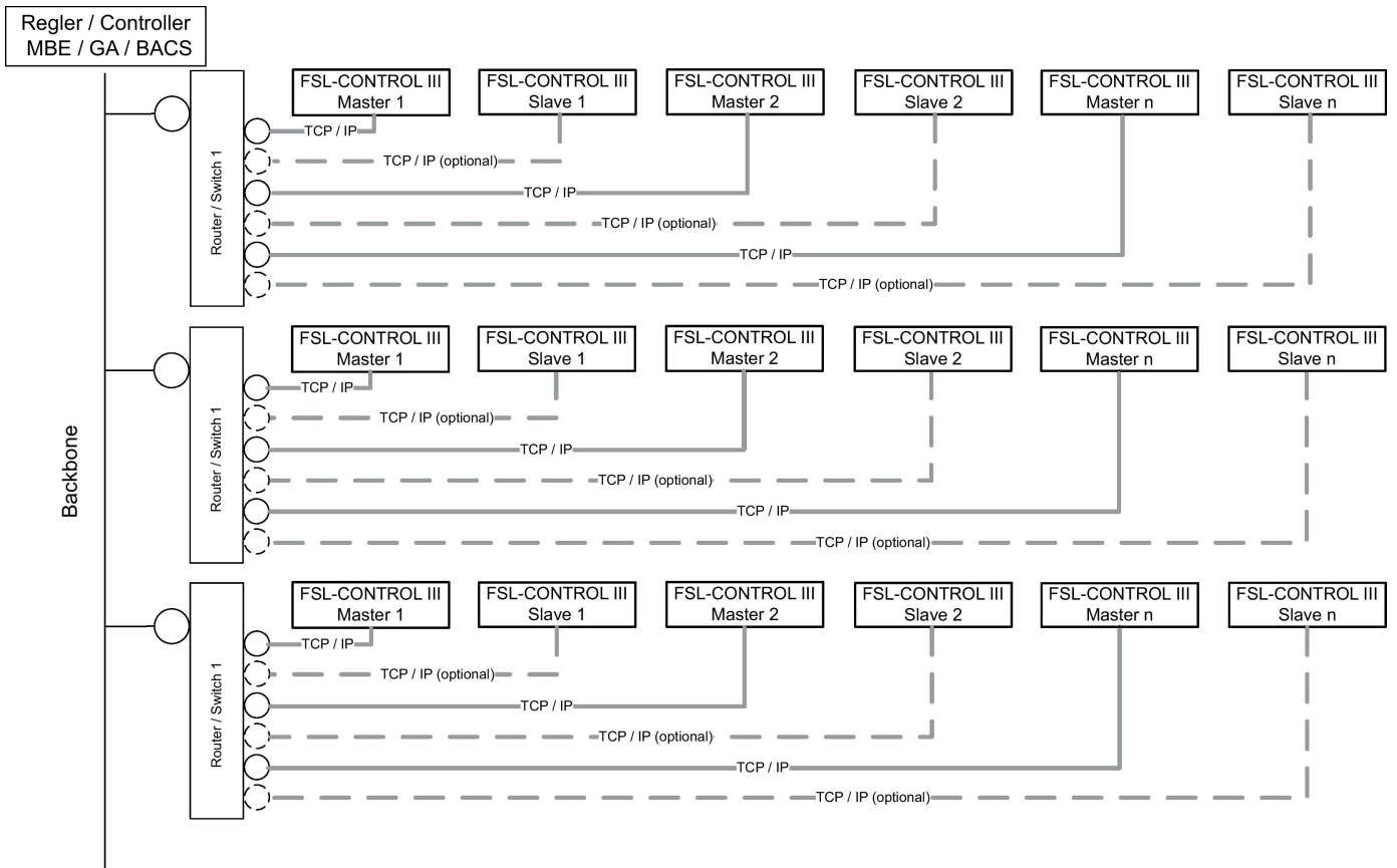
Abb. 22: FSL CONTROL III Netzwerkaufbau, Modbus TCP; BACnet IP
