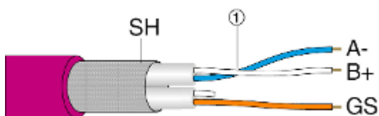
Abb. 17: Verdrahtung
