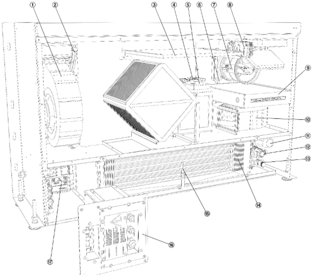
Abb. 41: Ersatzteile FSL-B-ZAB/SEK, Reglerbox herausgezogen
