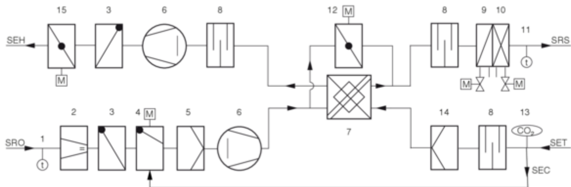
Abb. 3: Lüftungsschema ROOMAIR-B-ZAB/SEK
