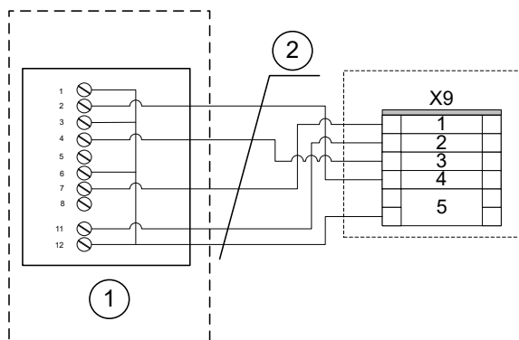
Abb. 9: Verdrahtung Raumbediengerät Thermokon, 5-stufig an Klemme X9
