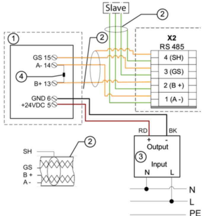
Abb. 8: Verdrahtung digitales Raumbediengerät Typ Schneider an Klemme X2
