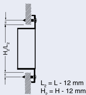
Fixação sem moldura de montagem Séries AT, VAT, AH, AE, AR, AGS.
