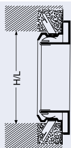
Grelha com fixação invisível através de molas e molduras ER Séries AT, VAT, AH, AR, AE Só para os tamanhos padrão L máx : 1225 mm e montagem em posição vertical.
