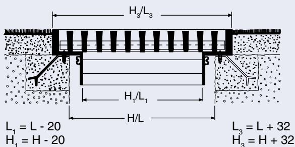
Série AF – Montagem com chumbadores A Grelha está fixada através de molas na sua moldura e deve ser retirada para a ajustagem do registro.
