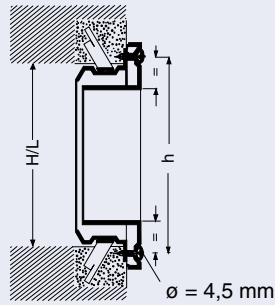
Grelha com parafusos aparentes Séries AT, VAT, AH, AE, AR, AGS h = H + 5 mm h = H + 10 mm (para a série AGS)
