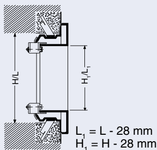
Grelha com fixação invisível através de PIN Séries AT, VAT, AH, AE Necessariamente com moldura de montagem “ER”.
