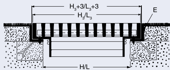
Série AF - Montagem com cantoneira interna (não faz parte de nosso fornecimento). A grelha neste caso pode ser retirada com sua moldura e registro.
