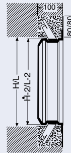
Molduras de montagem “ER” Os parafusos de fixação das grelhas podem ser aparentes ou invisíveis. Na montagem da moldura deve haver cuidado para evitar deformações da mesma.
